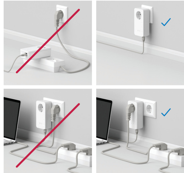
Rys.5: Optymalizacja przepustowości devolo Mesh
