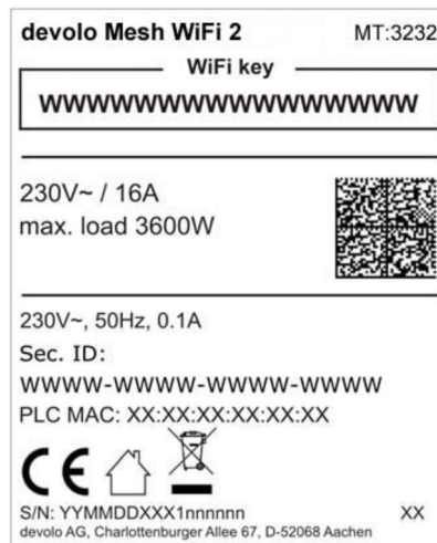
Afb. 4:andspecifieke identificatieplaatje
