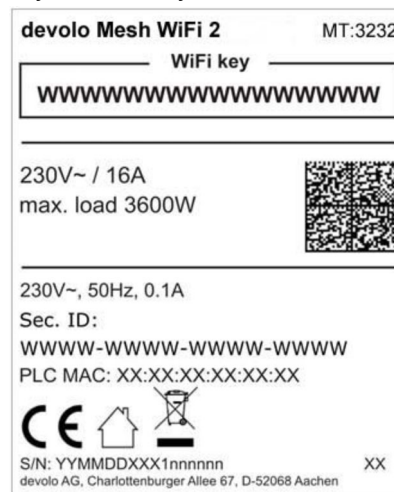
Rys. 4: Tabliczka znamionowa odpowiednia dla danego kraju
